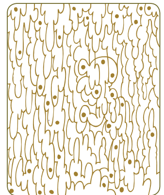
Lösung: Man erkennt in einer Tropfsteinhöhle beträchtliche Taschelnampe Gebilde in einer Tropfsteinhöhle.
